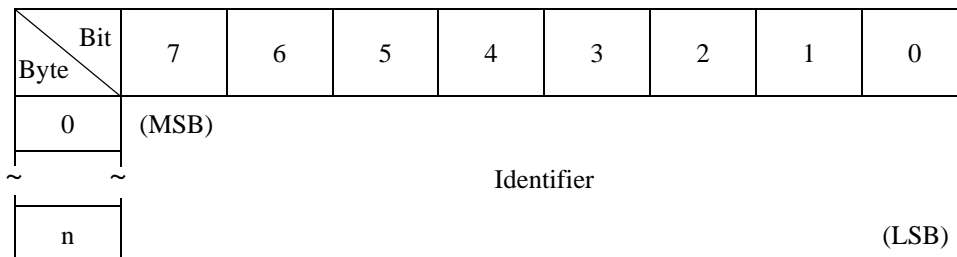
Figure 3.21 SET DEVICE IDENTIFIER: parameter list
