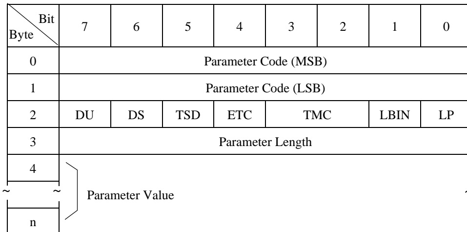
Figure 3.14 LOG SELECT command: log parameter
